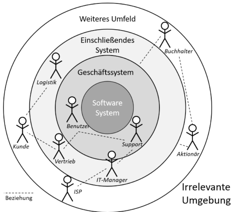
Abbildung 4.2 Alexanders Zwiebel-Modell
