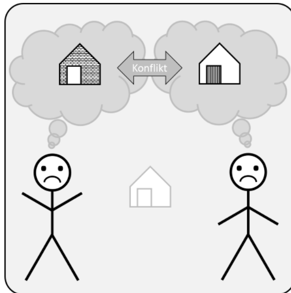
Abbildung 4.9 Ein Anforderungskonflikt
