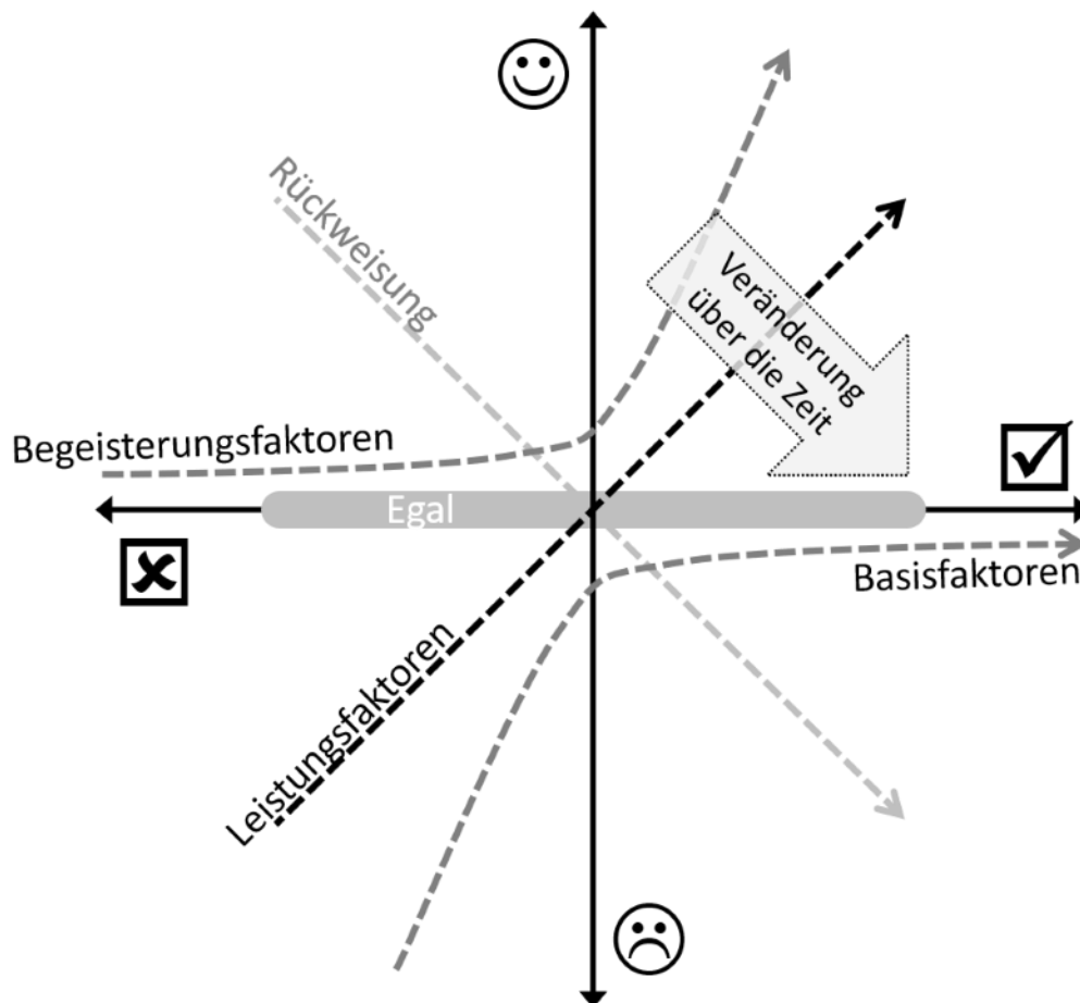
Abbildung 4.5 Das Kano-Modell
